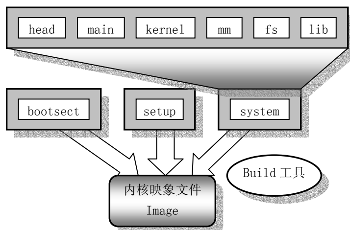
图 2.8 内核编译连接/组合结构
