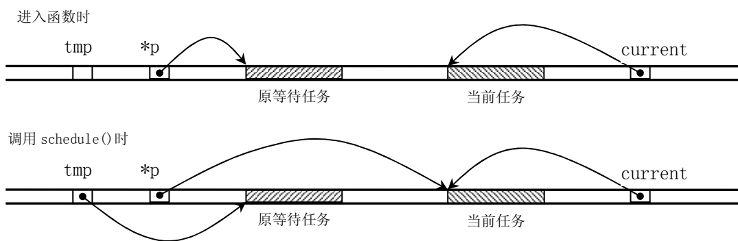
图 5.2 sleep_on() 函数中指针变化示意图。
