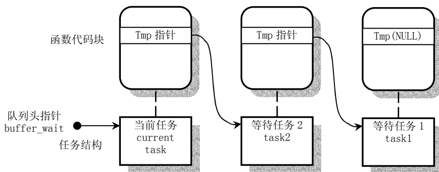
图 5.3 sleep_on() 函数的隐式任务等待队列。
