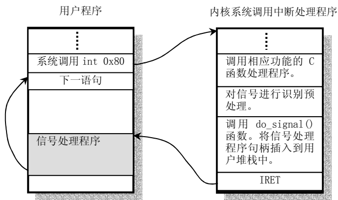
图 5.4 信号处理程序的调用方式。
