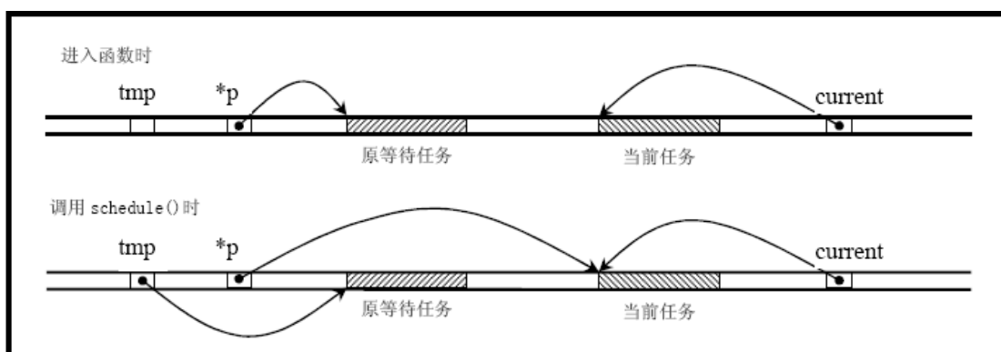
图 7.1 sleep_on 中指针变化图 (此图出自于《Linux0.11 完全注释》)
