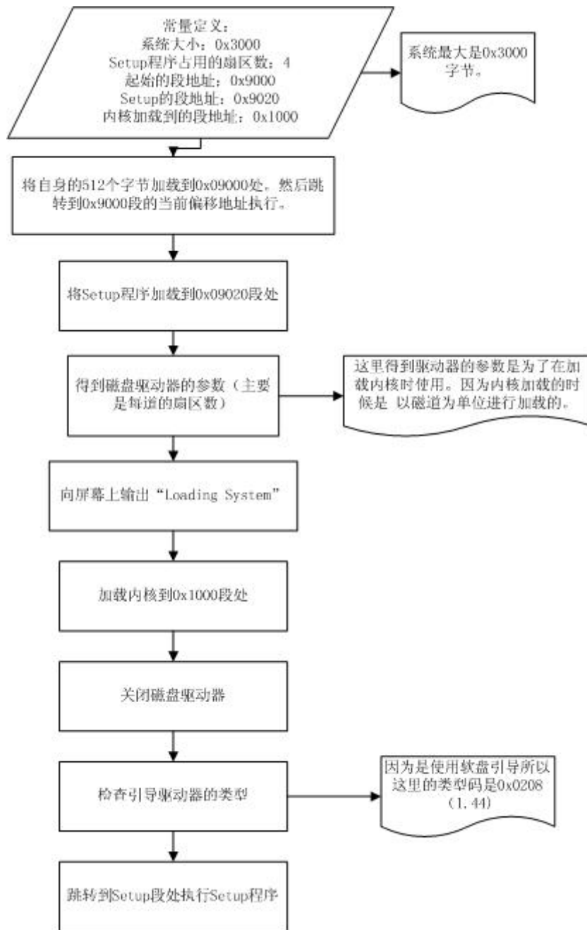
图 二.2bootsec.s 流程图
