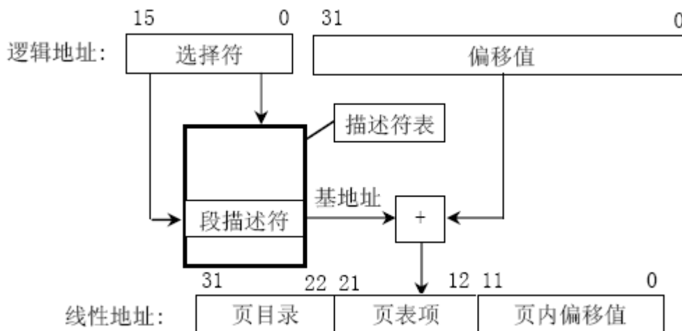
图 二.9 段变换示意图（出自于《Linux0.11 源码完全注释》）
